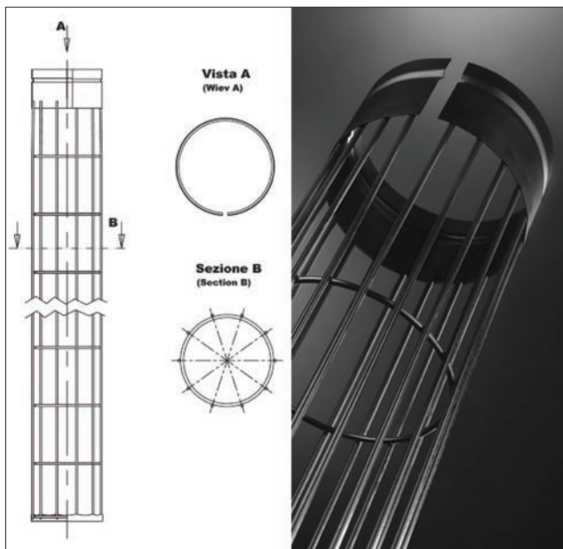
Figura 1 - Esempio di telaio filtro per montaggio sottopiastra (Mod. FB®). Figure 1 - An example of filter cage for mounting from below (Mod. FB®).
